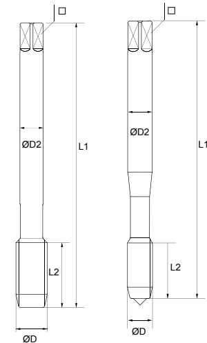
Shank: DIN 376
